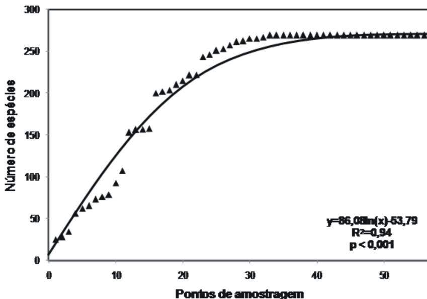
Figura 2. Curva espécie-área para os pontos de amostragem da vegetação da Serra da Canastra, Parque Nacional da Serra da Canastra (MG).
