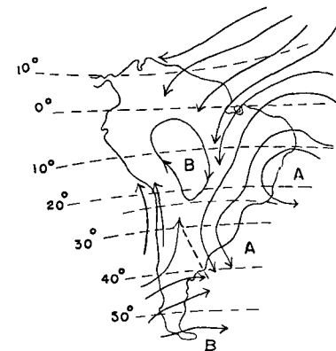
PRIMAVERA OUTUBRO - VENTOS MÉDIOS NÍVEL 500 M. Fig. 39
