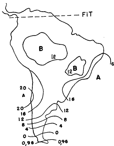
QUADRO DAS PRESSÕES MÉDIAS (OUTUBRO) PRIMAVERA
