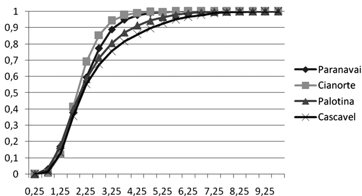
Gráfico 1 - P(V \leq v) = probabilidades empíricas de ocorrência de valores menores ou iguais à velocidade média diária do vento ( v ), para as cidades de Paranavai, Cianorte, Palotina e Cascavel
