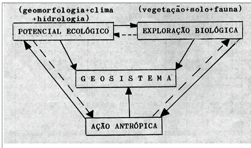
Figura 1: Classificação tipológica do geossistema bertrandiano.
