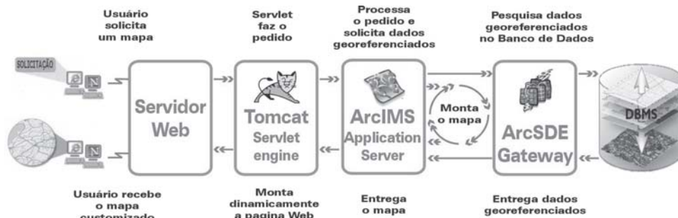
Figura 1 - Fluxo de solicitação e retorno de mapas, vigente na versão 2.0 do Atlas
