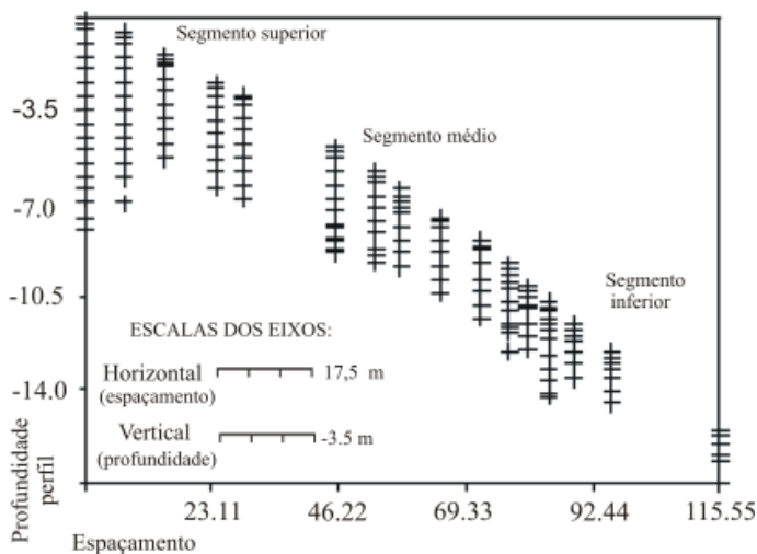
Figura 2 - Localização e distribuição das amostras ao longo da topossequência estudada. Os valores dos eixos vertical e horizontal correspondem respectivamente à profundidade e espaçamento lateral entre os furos de sondagem
