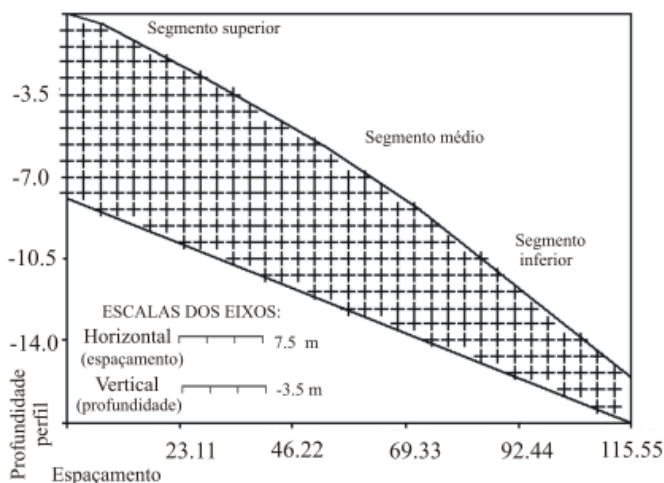
Figura 3 - Definição da Fronteira Convexa, segundo Yamamoto (1997b) para os 16 furos de amostras de solos dispostos ao longo da topossequência
