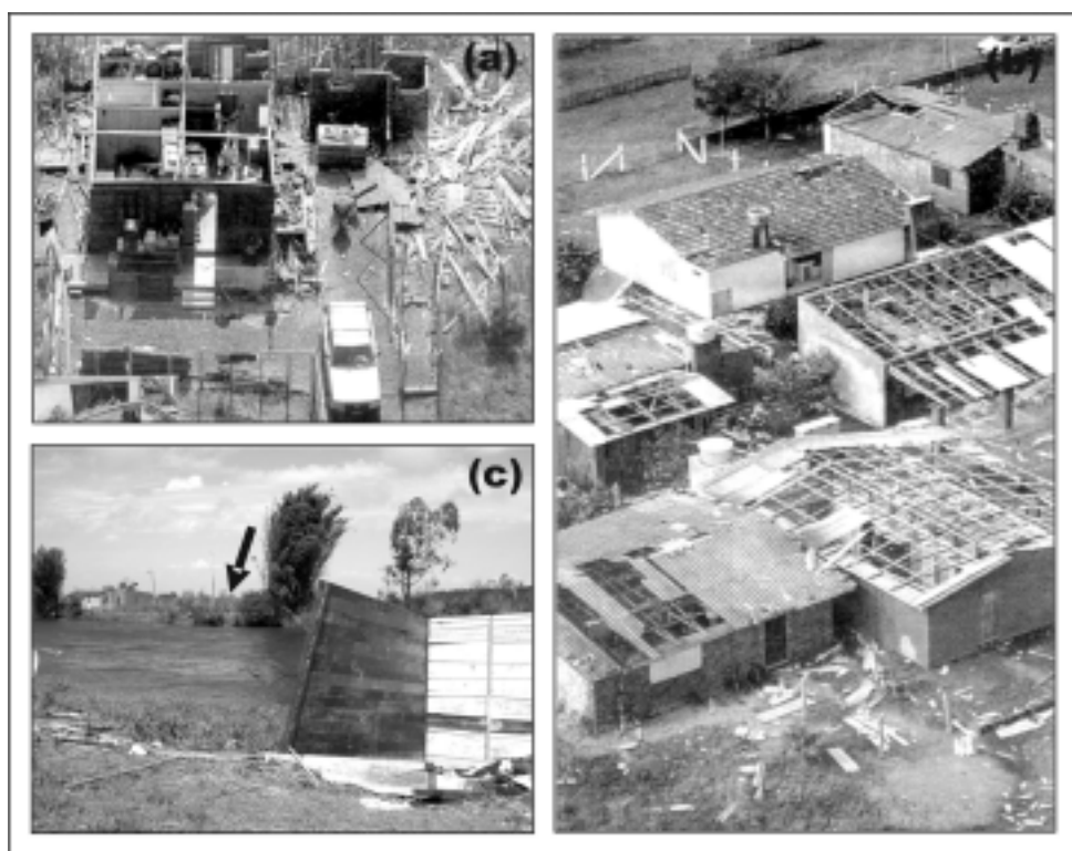
Figura 12 – Tipos de danos causados pela força dos ventos: (a e b) destelhamentos e destruição de generalizada de telhados; e (c) casa destruída, lançada pelos ventos sobre o rio Mampituba, divisor que separa os estados do Rio Grande do Sul e Santa Catarina
