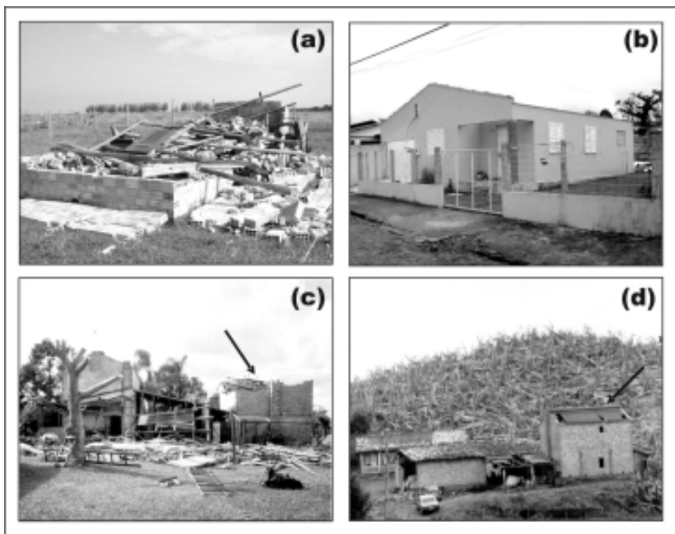
Figura 2 – Exemplo dos danos causados pelo Furacão Catarina sobre as edificações e suas respectivas classes de impacto: (a) Muito Alta; (b) Alta; (c) Média; e (d) Baixa
