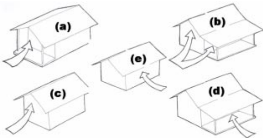
Figura 9 – Susceptibilidade das residências associadas à forma dos telhados e direção dos ventos
