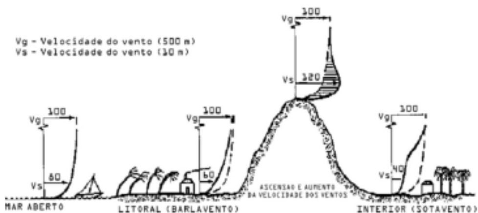
Figura 5 – Comportamento dos ventos típicos de um furacão em relação à topografia
