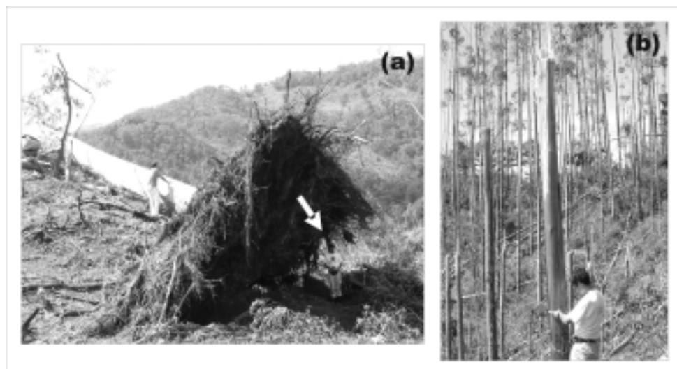
Figura 6 – Comportamento dos ventos canalizados em um vale sobre a vegetação: (a) nas encostas, a barlavento; e (b) próximo à crista, a sotavento
