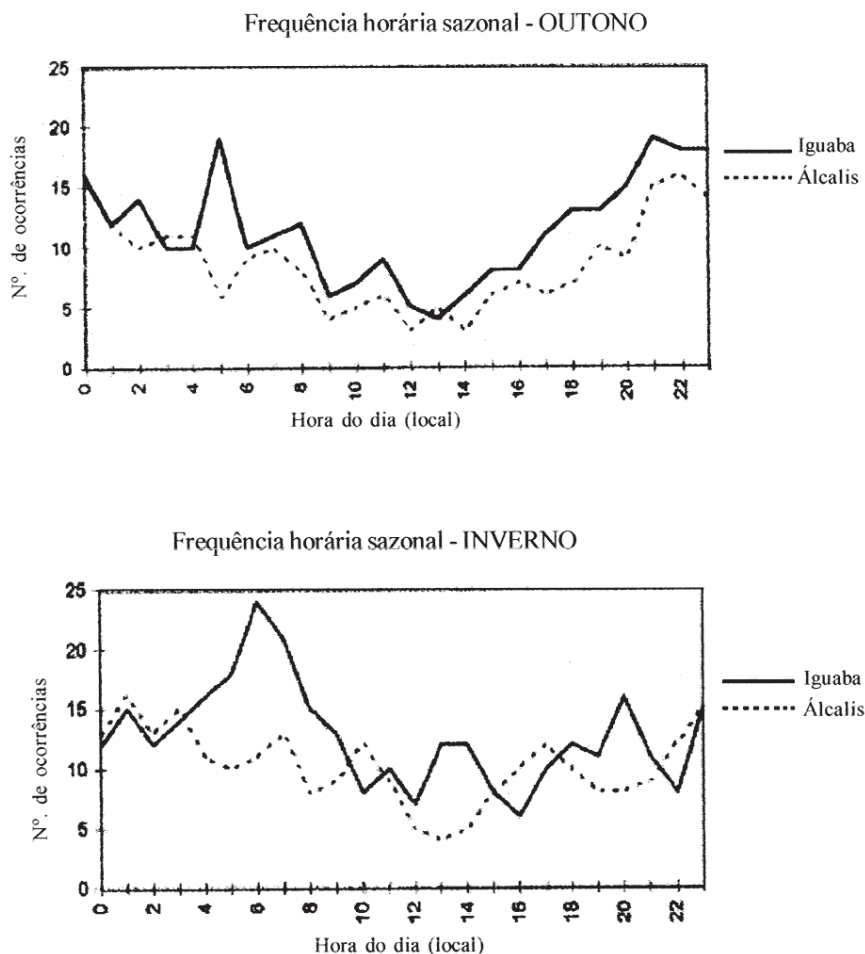
Figura 8B – Frequência horária sazonal de eventos de chuvas para as estações meteorológicas de Álcalis e Iguaba (Outono e Inverno)
