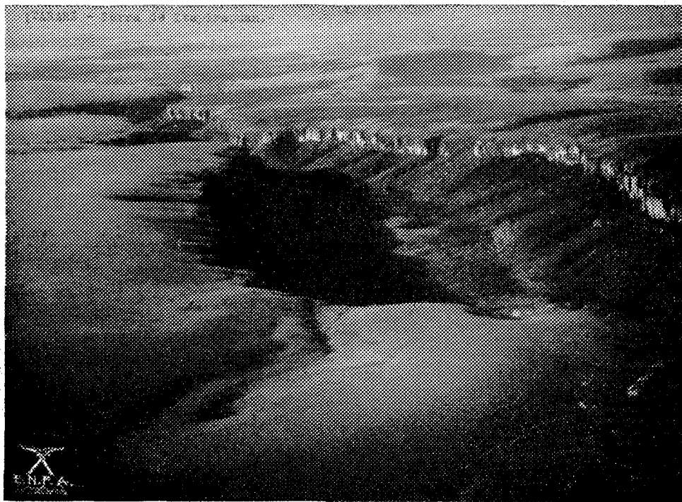
Aspecto do planalto meridional, em Itararé (São Paulo). Uma das faixas de terrenos sedimentares, que se sucedem no planalto, é constituída de arenitos devonianos, formando uma “cuesta” desde Faxina até as nascentes do Iguassú, a qual no Paraná recebe o nome de Serrinha (segundo degrau do planalto). O rio Itararé entalha profundamente essa faixa, formando um belo “canyon”.
