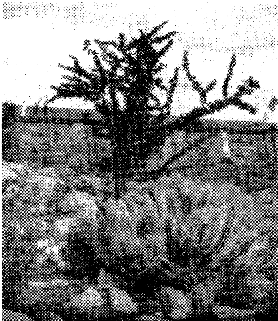
Aspecto típico da região semi-árida do Nordeste, com sua vegetação xerófila (caatinga). Foto tirada nas proximidades da cachoeira de Paulo Afonso. A comparação com a fotografia anterior mostra o contraste entre a Amazônia super-úmida e o Nordeste semi-árido.
