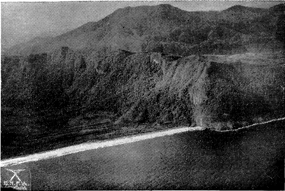
Trecho do litoral meridional em que a Serra do Mar é diretamente batida pelo oceano. Foto da ponta da Juréia, no município de Iguape (São Paulo).
