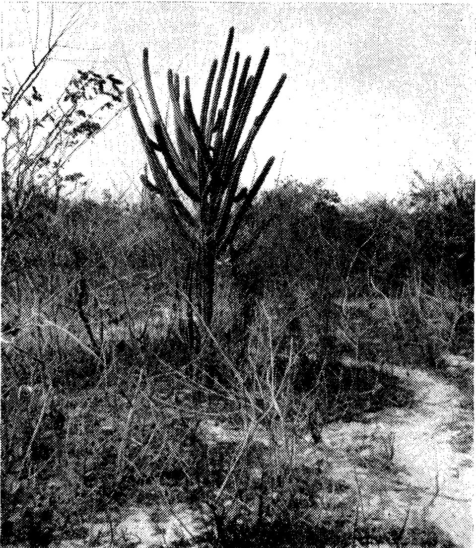
Caatinga no Estado do Piauí. vegetação xerófila, típica do Nordeste brasileiro.
