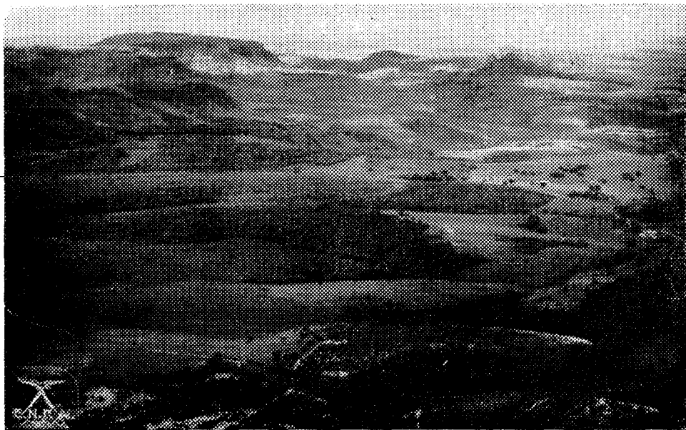
Aspecto da serra de Botucatú, em Itatinga (São Paulo). No planalto meridional do Brasil a sucessão das camadas sedimentares é marcada frequentemente por escarpas ("cuestas"). A "cuesta" de Botucatú assinala a passagem dos arenitos permianos para os arenitos triássicos, capeados por derrames basalto-diabásicos.
